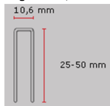
Agrafes N / G16
